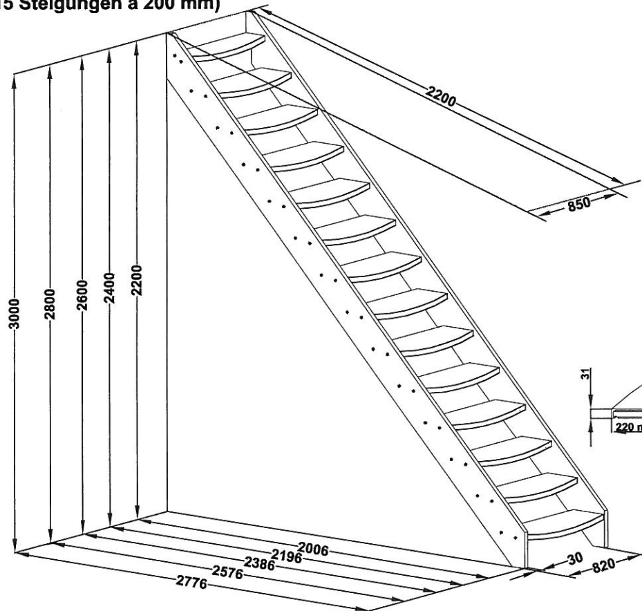
Planung Geradläufige 14 Stufen ( 15 Steigungen a 200 mm)
